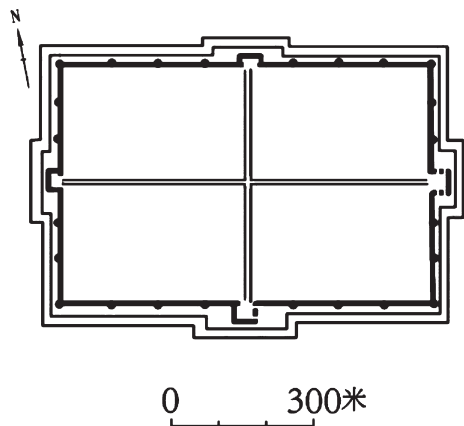
〔图二〕黑城城址平面图
